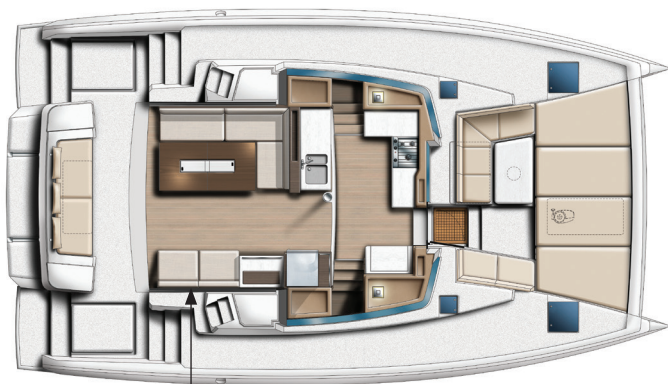
Nacelle (Fauteuils en option) / Saloon (Optional armchairs)
