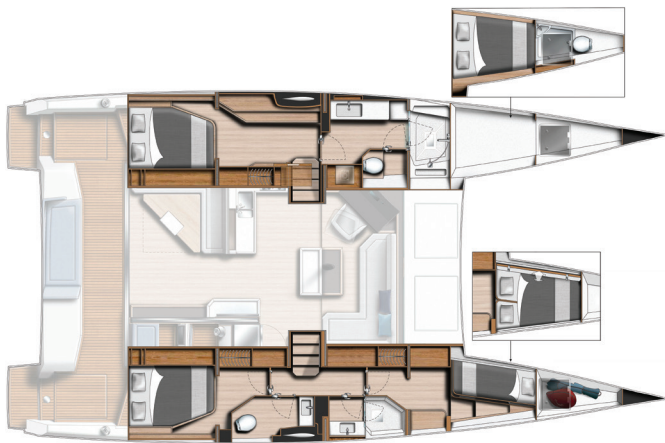
Version propriétaire 3 Cabines / 2 sdb + skipper ( Option )
