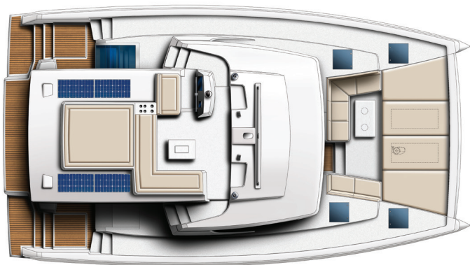
Pont et Flybridge / Deck and Flybridge Pont teck en option / Optional Teak deck
