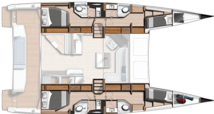
Version 4 Cabines / 4 sdb
