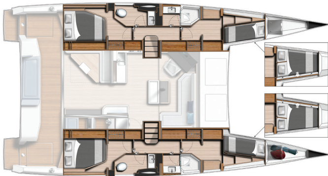
Version 4 Cabines / 2 sdb
